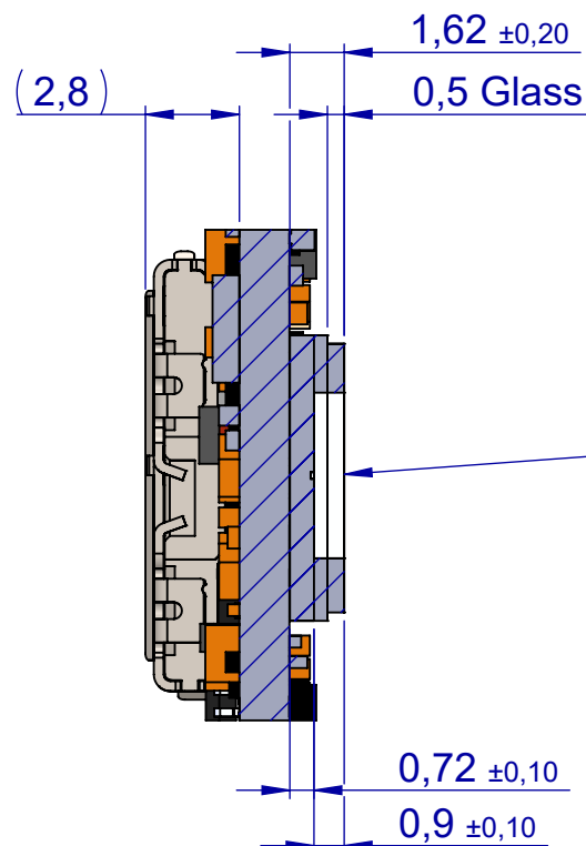
SCHNITT B-B MAßSTAB 4:1
